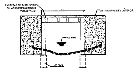
CORTE-BB' Escala 1/50
