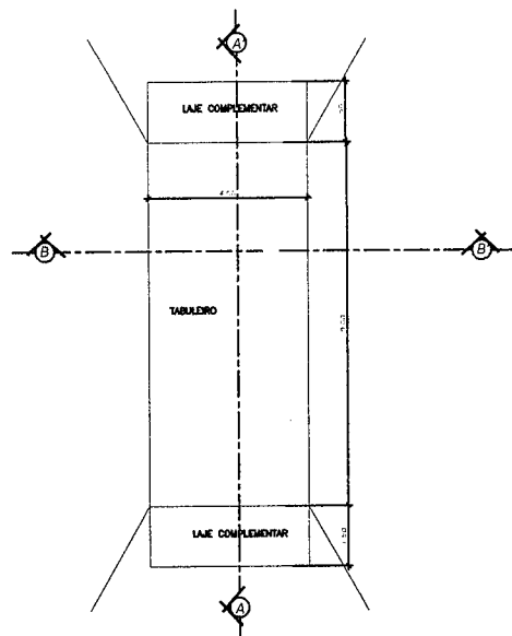
PLANTA BAIXA - TABULEIRO Escala 1/100
