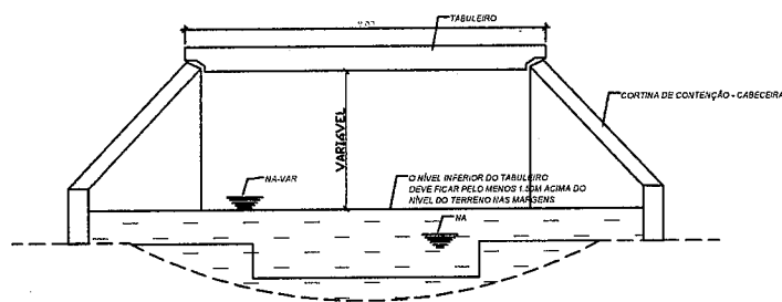
VISTA LATERAL Escala 1/100
