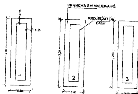
EQ. 03 BANCOS VISTA SUPERIOR Escala -----1:50
