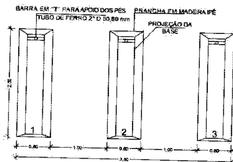
EQ. 04 PRANCHAS PARA EXERCÍCIOS ABDOMINAIS VISTA SUPERIOR Escala -----1:50
