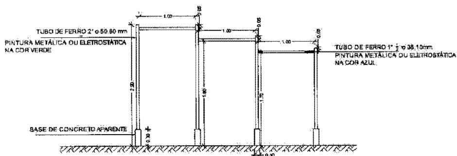
EQ. 05 BARRAS ASSIMÉTRICAS HORIZONTAIS ELEVÇÃO Escala -----1:50
