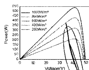
Curva de Potência-Tensão
