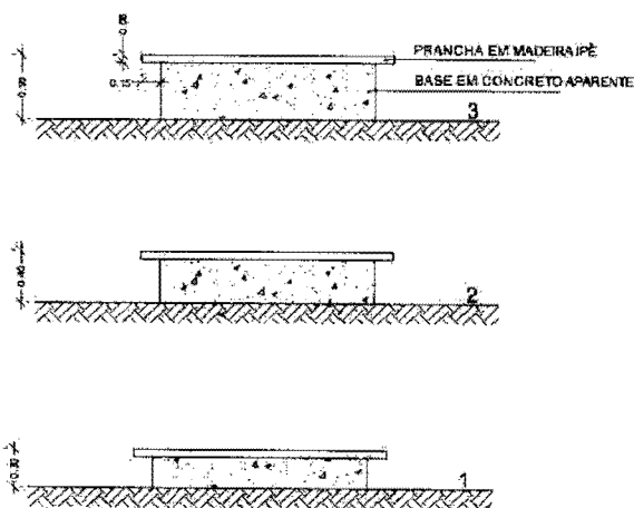
EQ. 03 BANCOS ELEVACÃO Escala: 1:50
