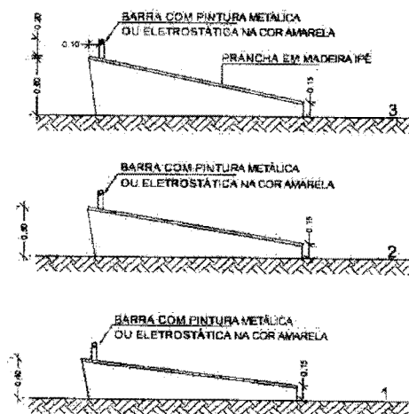
EQ. 04 PRANCHAS PARA EXERCÍCIOS ABDOMINAIS ELEVÇÃO Escala ----- 1:50
