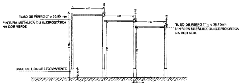
EQ. 05 BARRAS ASSIMÉTRICAS HORIZONTAIS ELEVÇÃO Escala -----1:50
