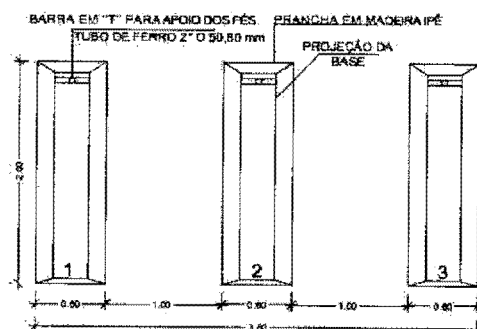
EQ. 04 PRANCHAS PARA EXERCÍCIOS ABDOMINAIS
