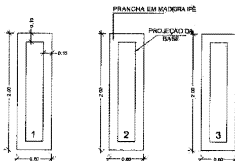
EQ. 03 BANCOS VISTA SUPERIOR Escala: 1:50
