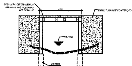
CORTE-BB' Escala 1/50
