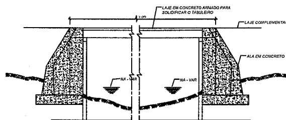
CORTE-AA' Escala 1/50
